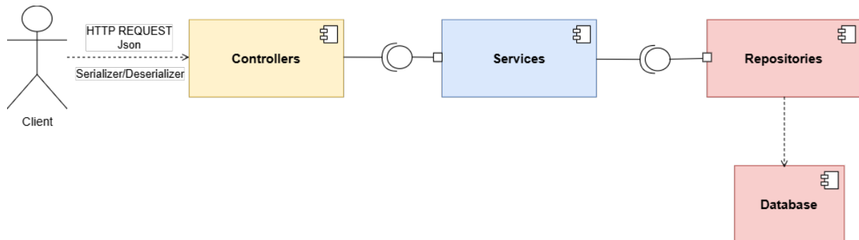
Figura 14: Schema architetturale 2 - Component Diagram del backend
